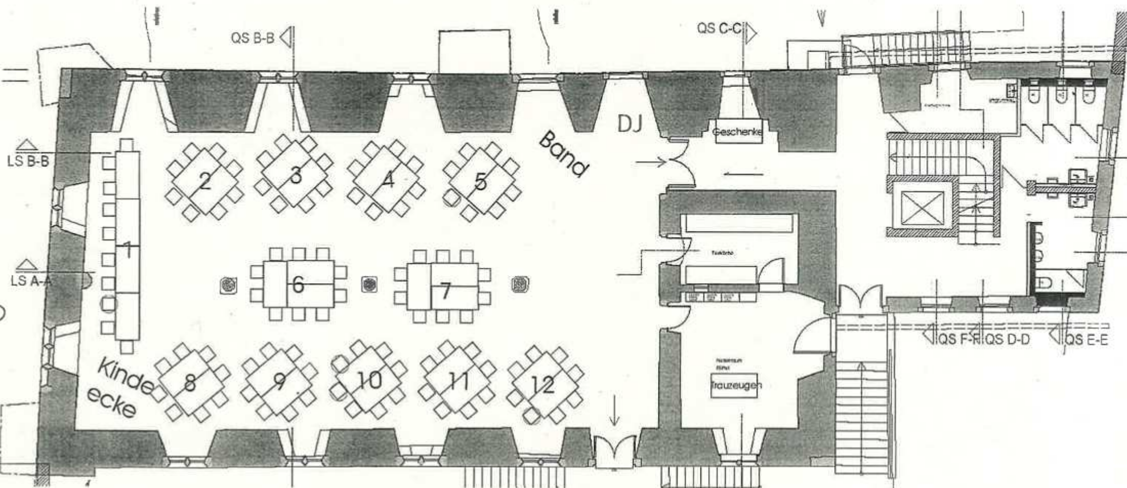
Grundriss EG 1:50
